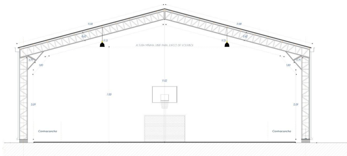
Imagen Proyecto de Construcción de Cubierta Multicancha Escuela Alto Pangue
